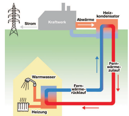
Das Prinzip der Fernwärme
